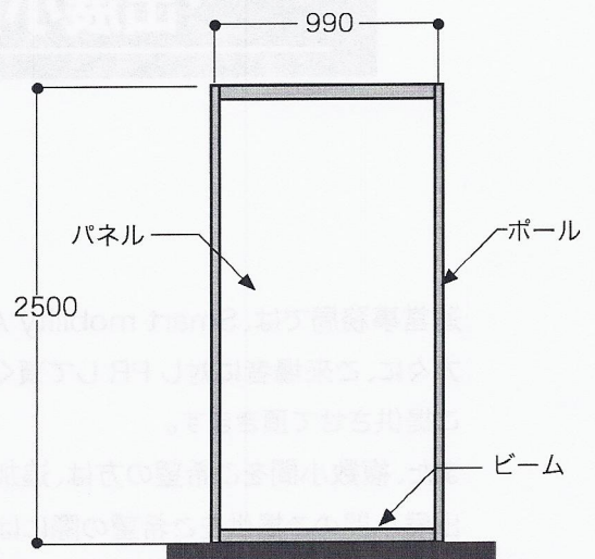
システムパネルの名称
